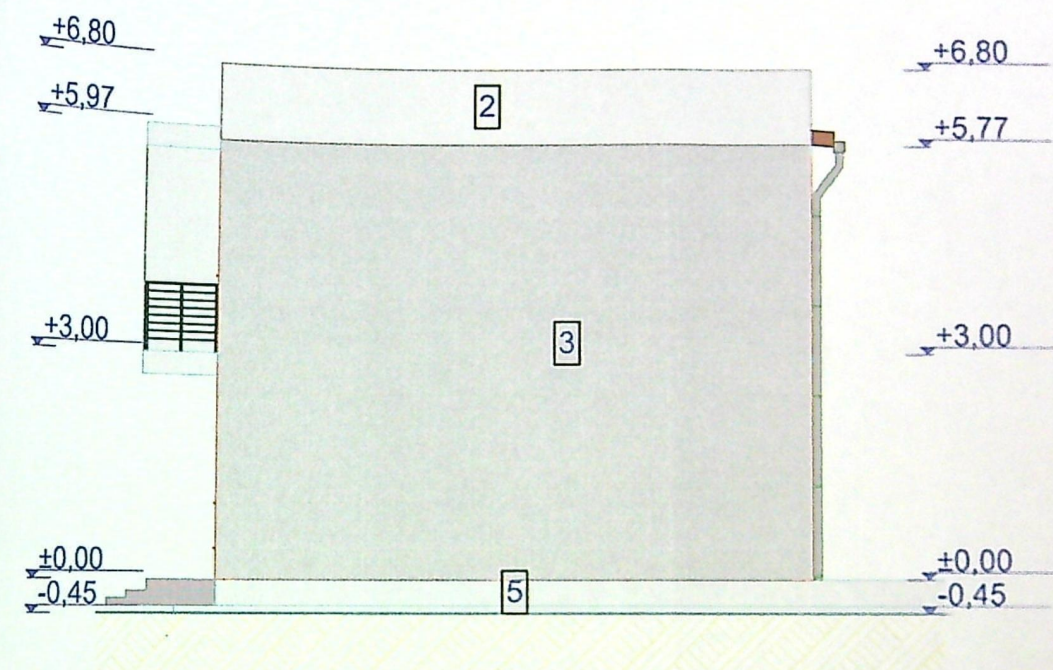
FATADA DREAPTA scara 1:100
