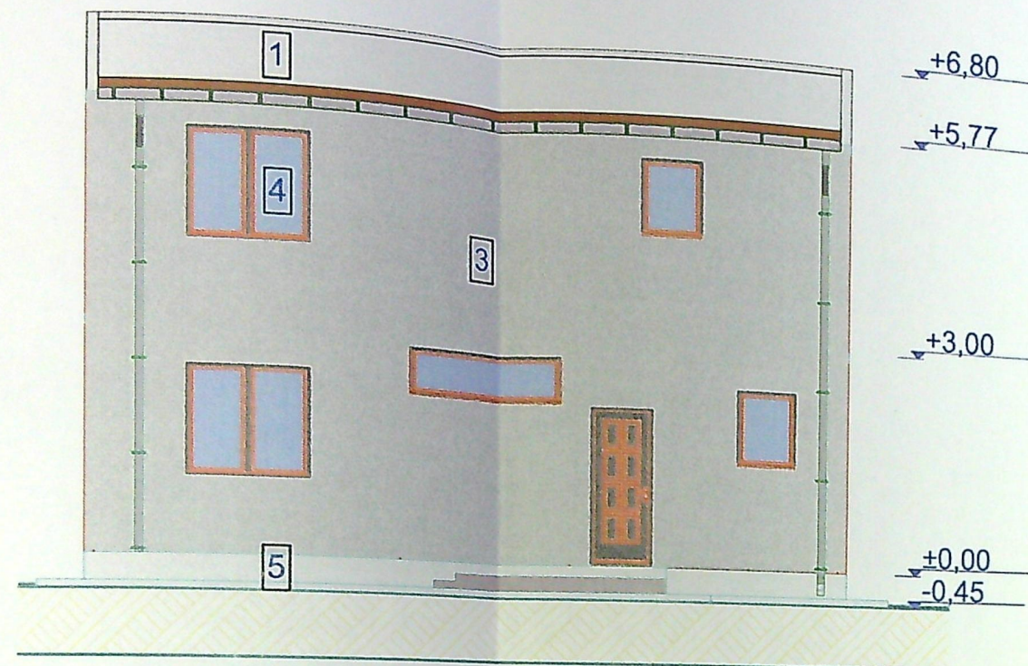
FATADA POSTERIOARA scara 1:100
